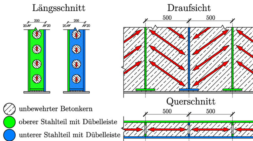
Abbildung 3: Vereinfachte Darstellung des Tragmechanismus der SCSC-Platte
